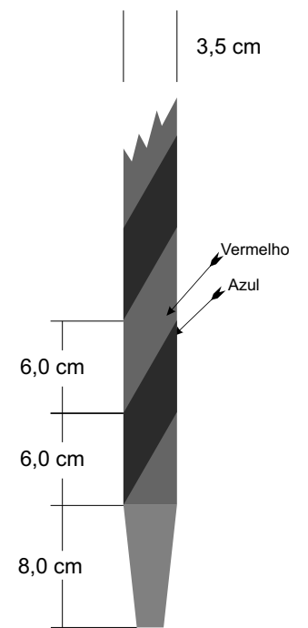
Conto de aço inoxidável (extremidade inferior da base)
